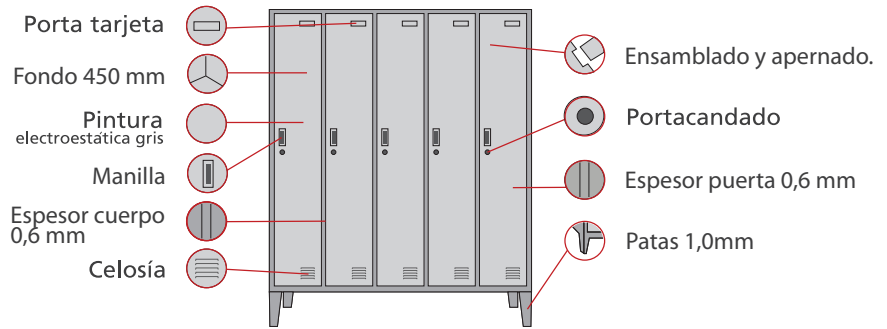
PUERTA: tirador y portacandado metálico
